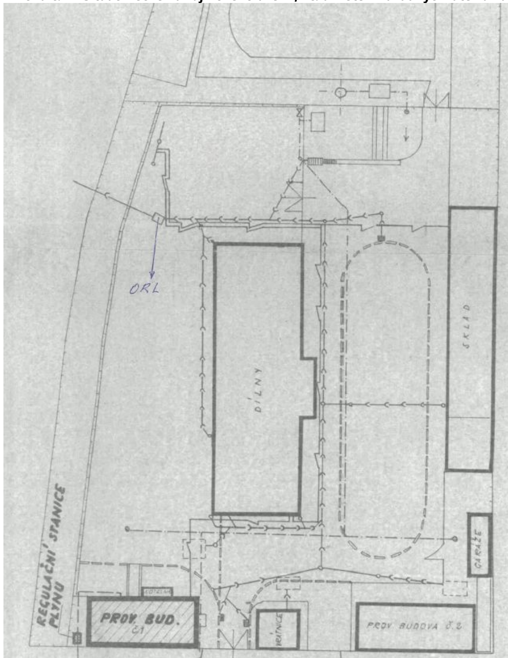
Příloha č. 1 Situační schéma zájmového území, vč. umístění závadných látek a kanalizace
